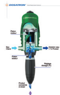
SÉRIE D8 GL 500 l/h à 8 m 3 /h
